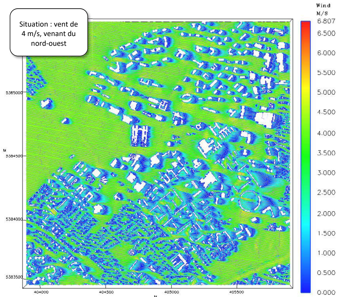
Figure 16 : lignes de courant et vitesse du vent à 2 m au-dessus du sol
