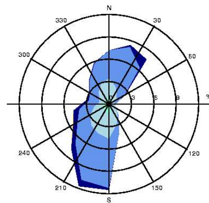
Figure 8 : rose des vents générale – 2020 à 2022
