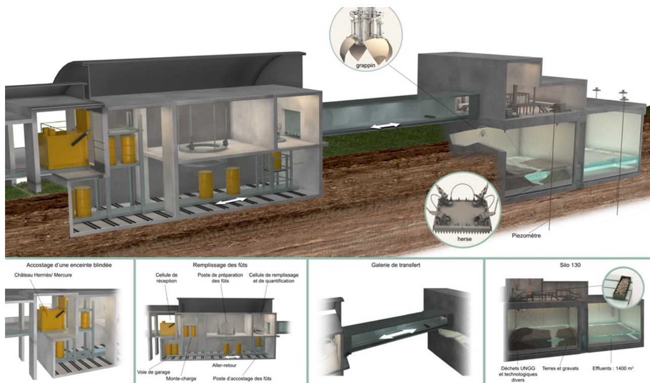
Schéma de reprise et conditionnement des déchets du Silo 130
