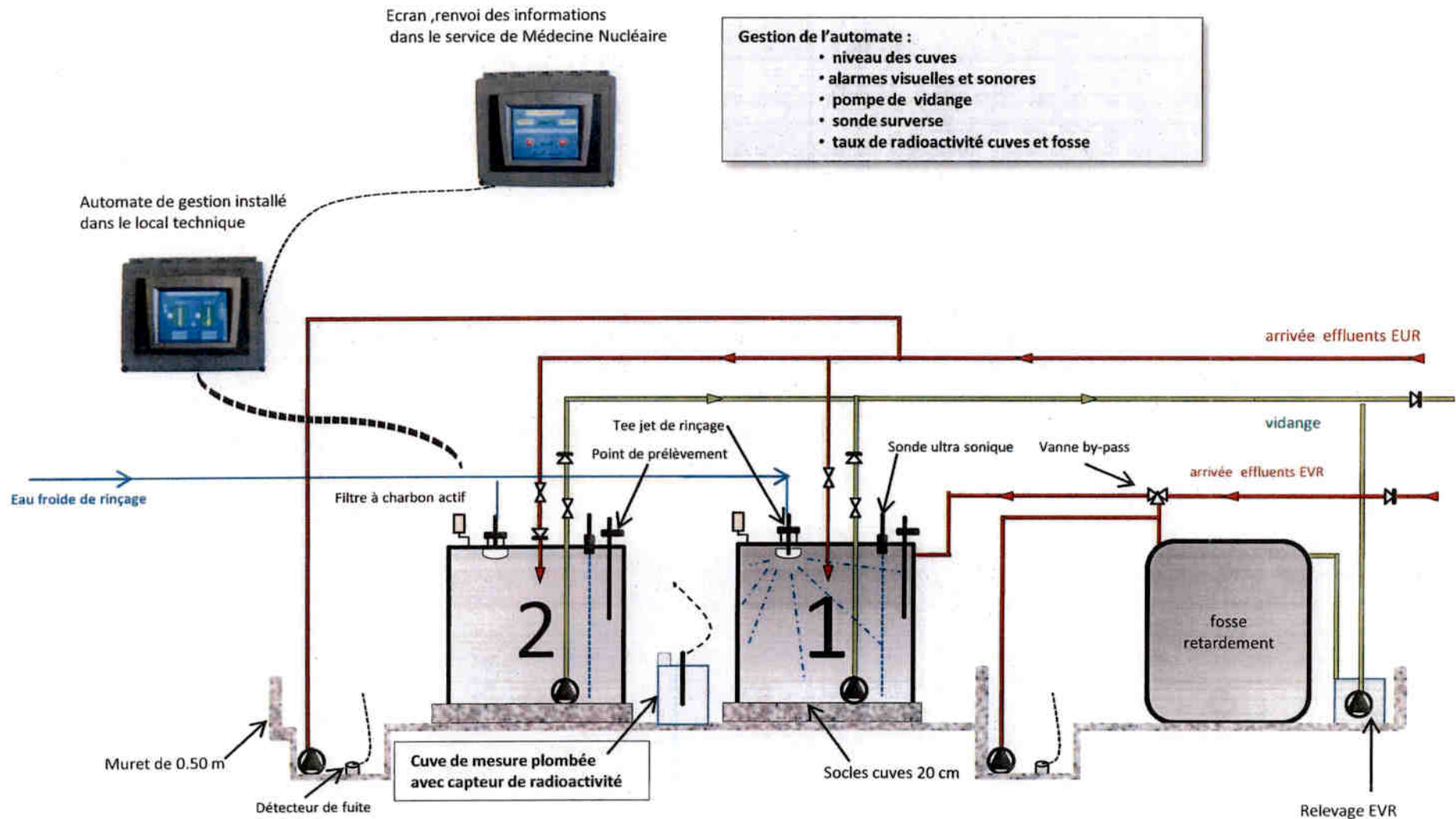
Schéma de principe installation de cuves pour l'entreposage et le traitement de décroissance d'effluents radioactifs du CH de Mont de Marsan
